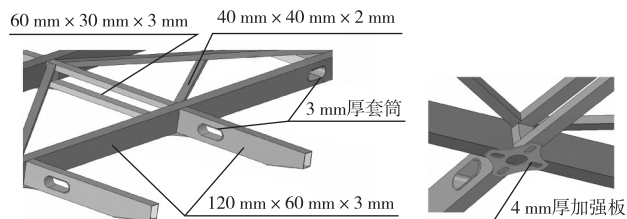
图2 单层矩形钢方案及局部位置结构
